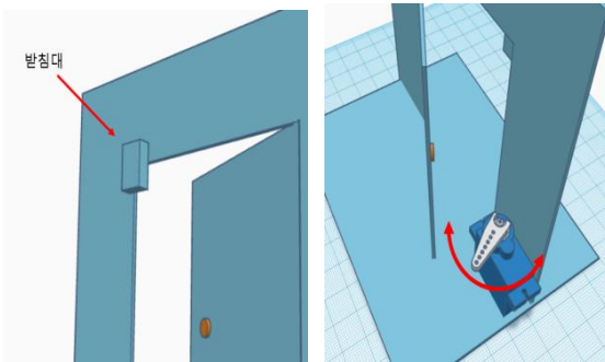
서보모터를 사용한 도어락
